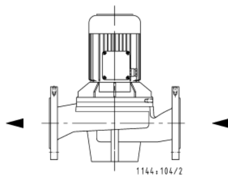
Вертикальный монтаж
