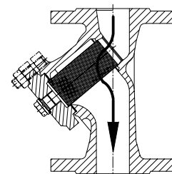
Вертикальная установка
